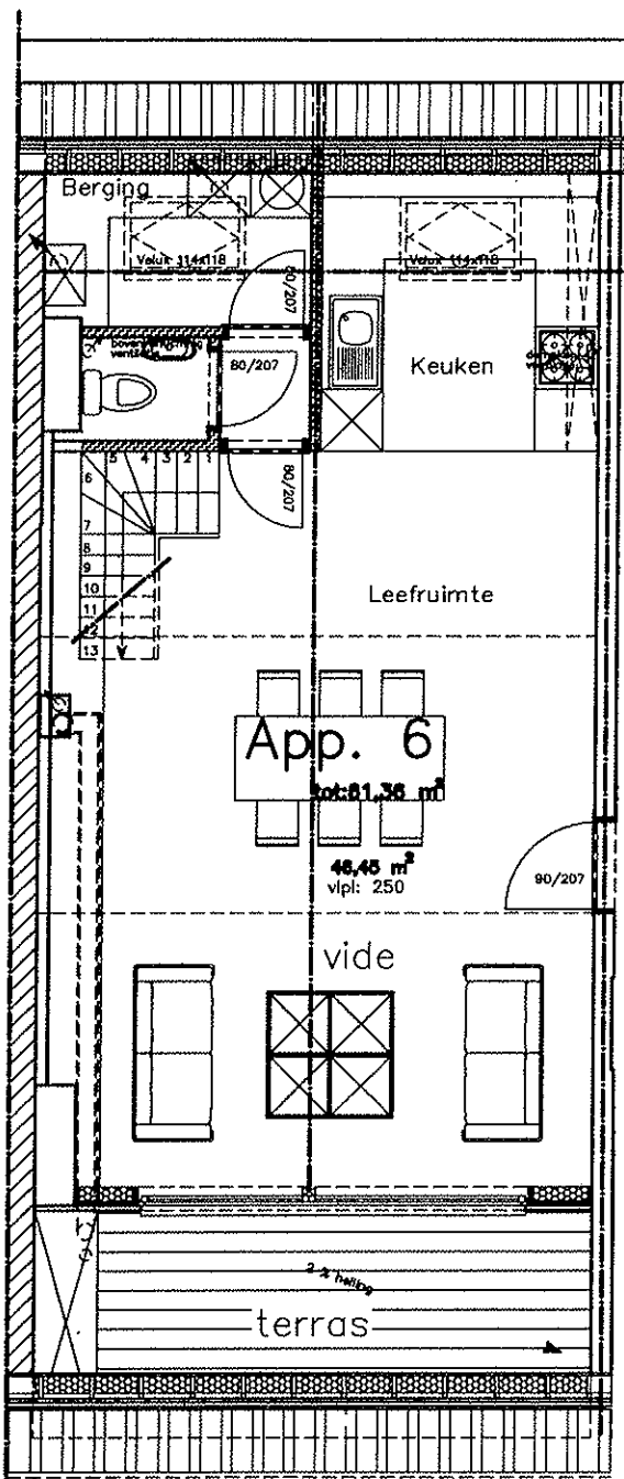
3 e VERDIEPING
